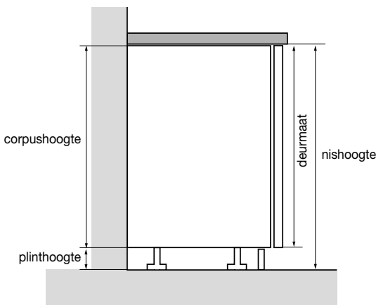
Inbouw situatie onder werkblad
