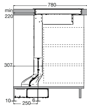
ZIJAANZICHT
