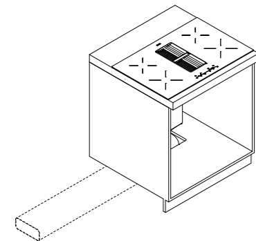
UITVOERING 2, LINKERUITLAAT (MIDDENSTUK GEDRAAID)
