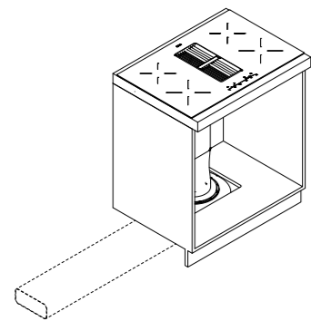
UITVOERING 1, LINKERUITLAAT
