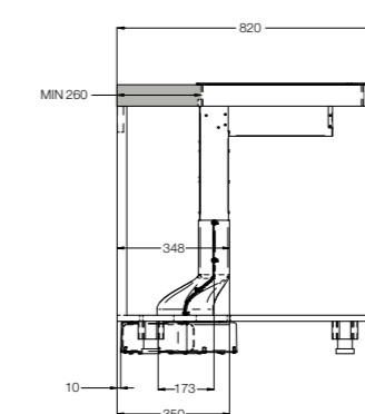
ZIJAAZICHT
