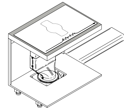
UITVOERING 2, RECHTERUITLAAT
