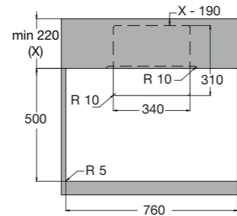
BOVENAANZICHT
